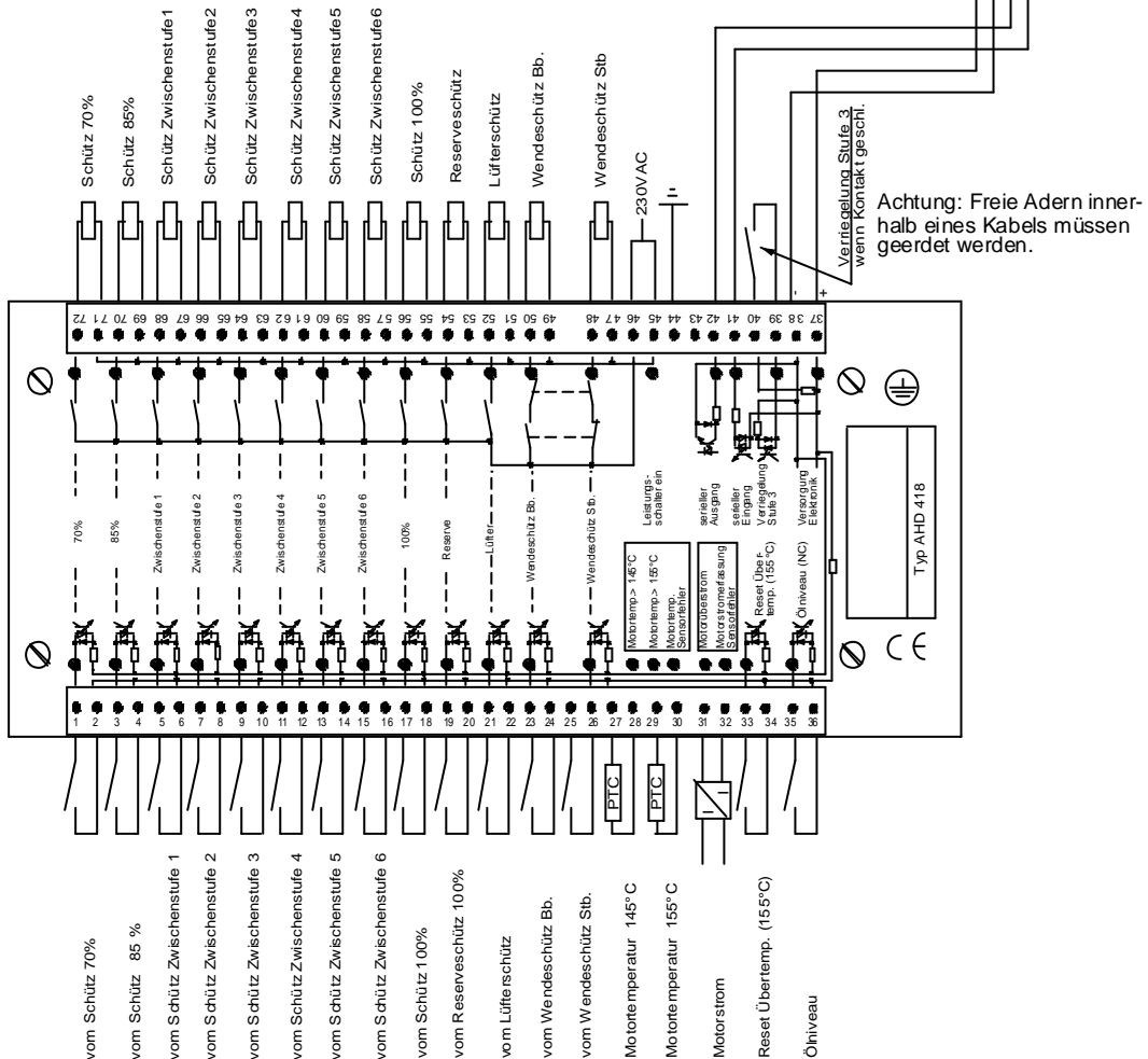
zentrales Steuermodul AHD 418 im Bugstrahlruderraum
