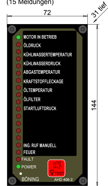
Einbaugehäuse (Tafelausschnitt 131 x 61mm)
