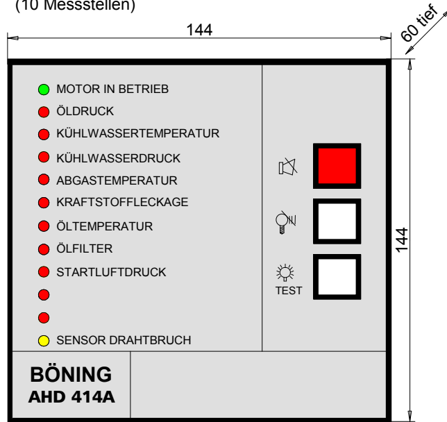
Einbaugehäuse für Tafelausschnitt 138mm x 138mm
